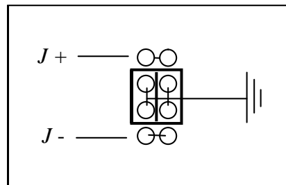
Рис. 9 Снятие заземления с выходных клемм источника
