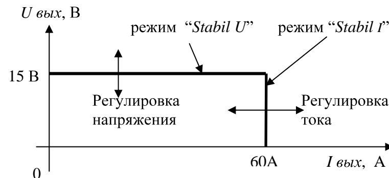
Рис. 4. Вольтамперная характеристика источника питания
