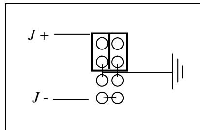
Рис. 8 Заземление плюсовой клеммы
