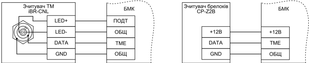
Рисунок 4 - Схема підключення зчитувача ключів ТМ (зліва) та зчитувача Proximity брелоків (зправа)
