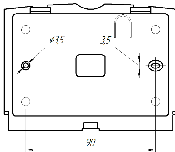
Рисунок В.2 – Установчі розміри клавіатури
