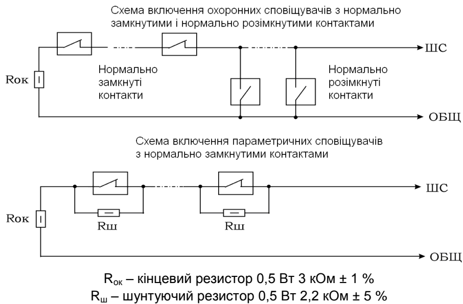
Рисунок 3 – Схеми включення сповіщувачів
