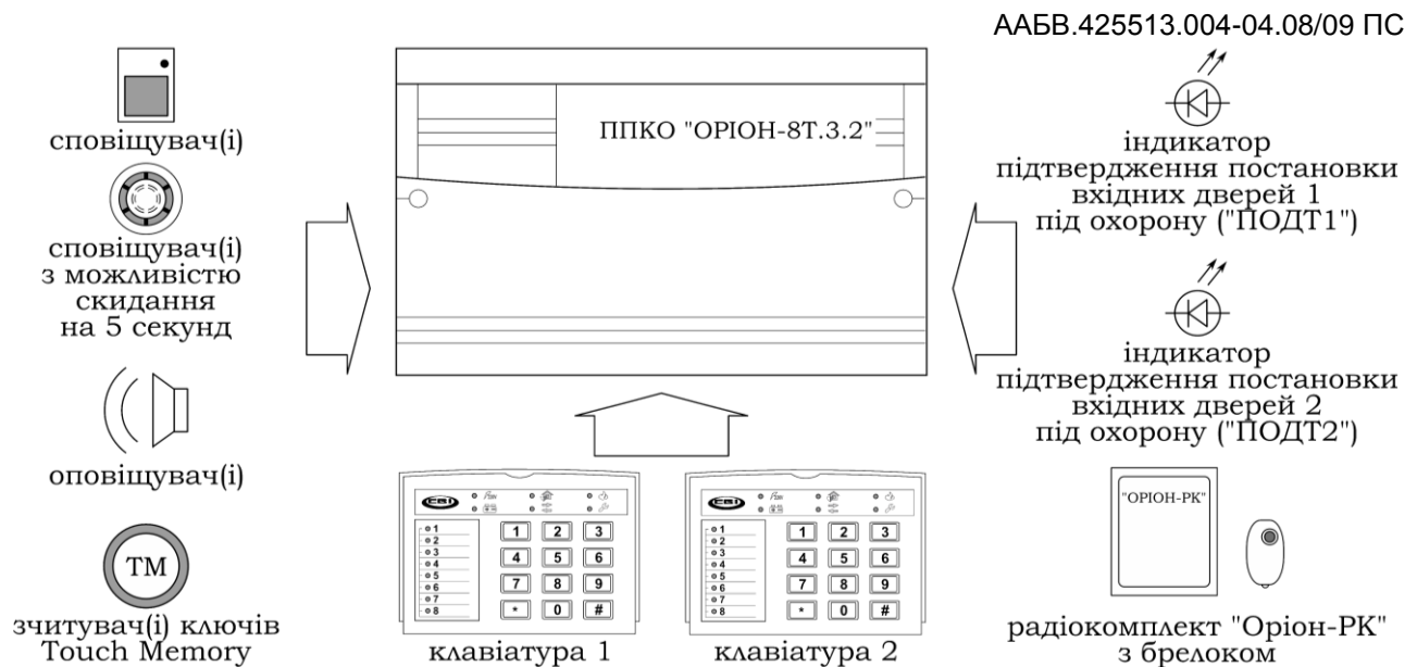
Рисунок 2 – ППКО «Оріон-8Т.3.2» в повному складі
