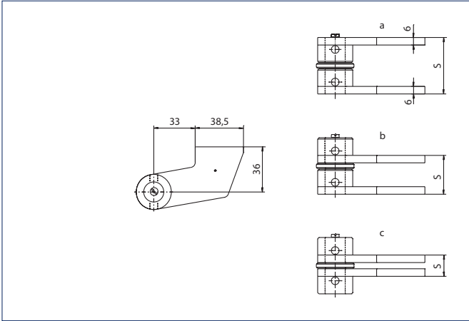
Верхняя поворотная опора (модель ЕК)
