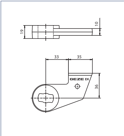
Нижняя поворотная опора (модель ЕК)
