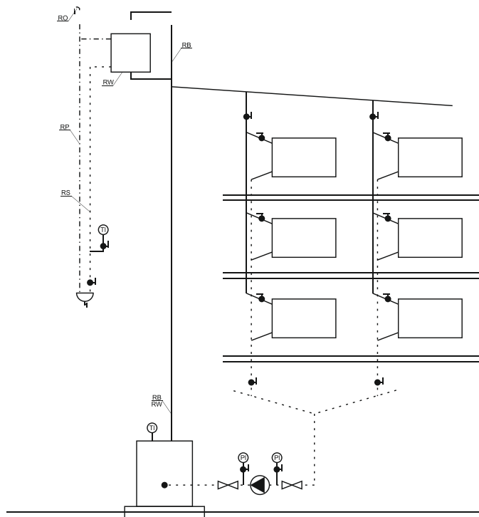
Схема інсталяції водяного обігріву, з одним котлом або теплообмінником, верхнім підключенням, насос замонтований на поверненні.
