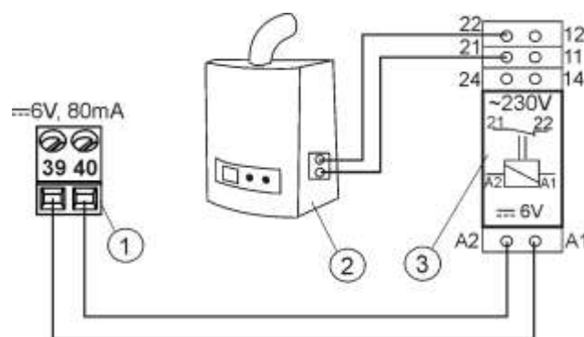
Мал. 23. Приклад схеми системи підключення резервного котла до контролера, де: 1-модуль B, 2-резервний котел (для газу), 3-конектор RM 84-2012-35-1006 і колодка GZT80 RELPOL.
