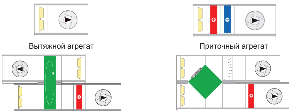
Агрегат с вращающимся теплообменником Агрегат с перекрестно-точным теплообменником
