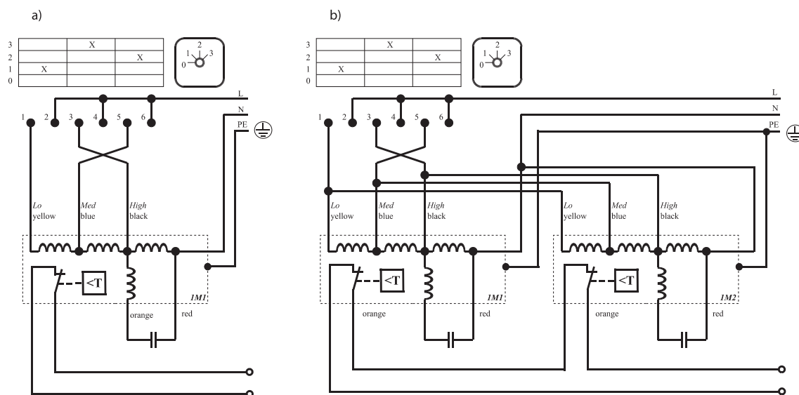
Рис. 23 Схема подключения двигателя в агрегатах VS 10 и VS 15
