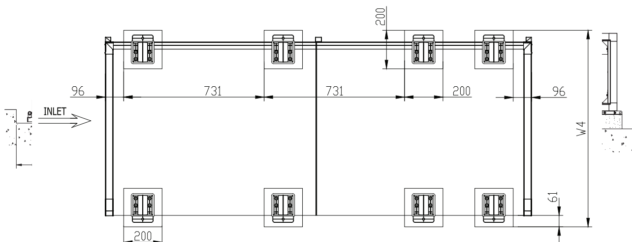
Рис. 13.d. Дополнительные опоры установки, оснащенной опорными подставками.
