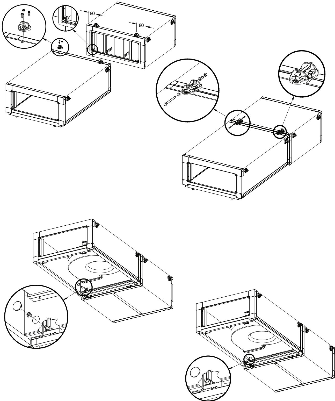
Рис. 8b. Соединение секции шумоглушения с секцией вентилятора.
