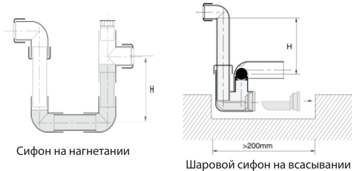
Рис. 20 Переливные сифоны
