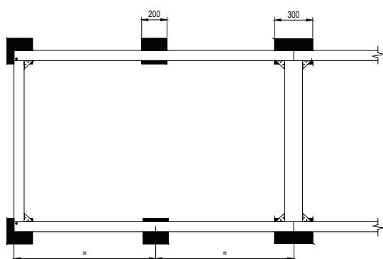
Рис.13 Местные подпорки рам блоков агрегатов
