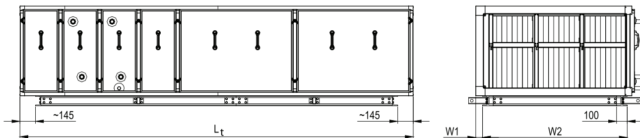
Рис. 12c. Транспортировочная рама (VS 21-150), изготовленная из литого профиля.
