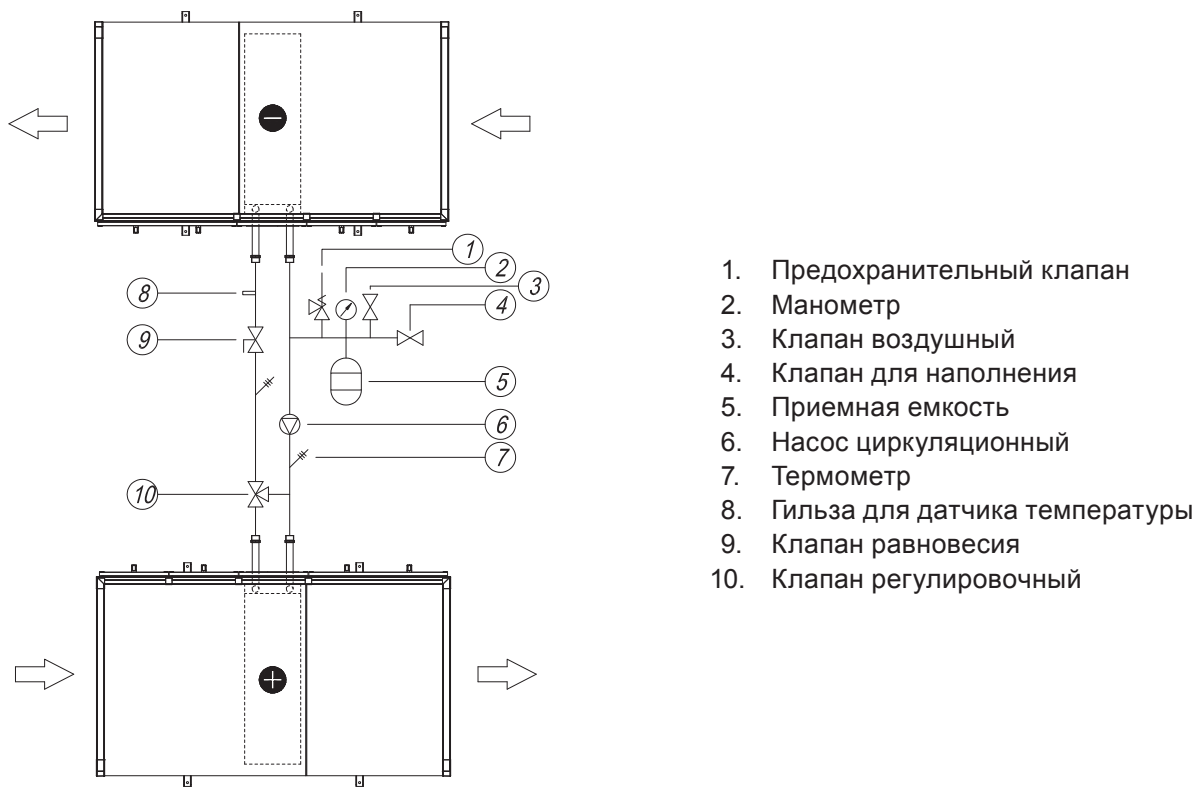
Рис.19 Пример подключения теплообменников
