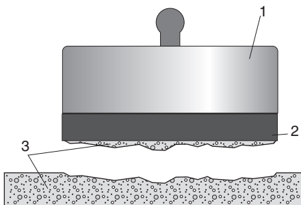
Рис.3 Отрыв по основанию (когезия основания)
