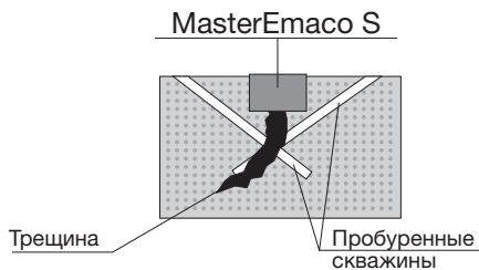
Рисунок 1. Примерная технология инъекции трещин
