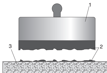
Рис.4 Отрыв по ремонтному материалу (когезия ремонтного материала)
