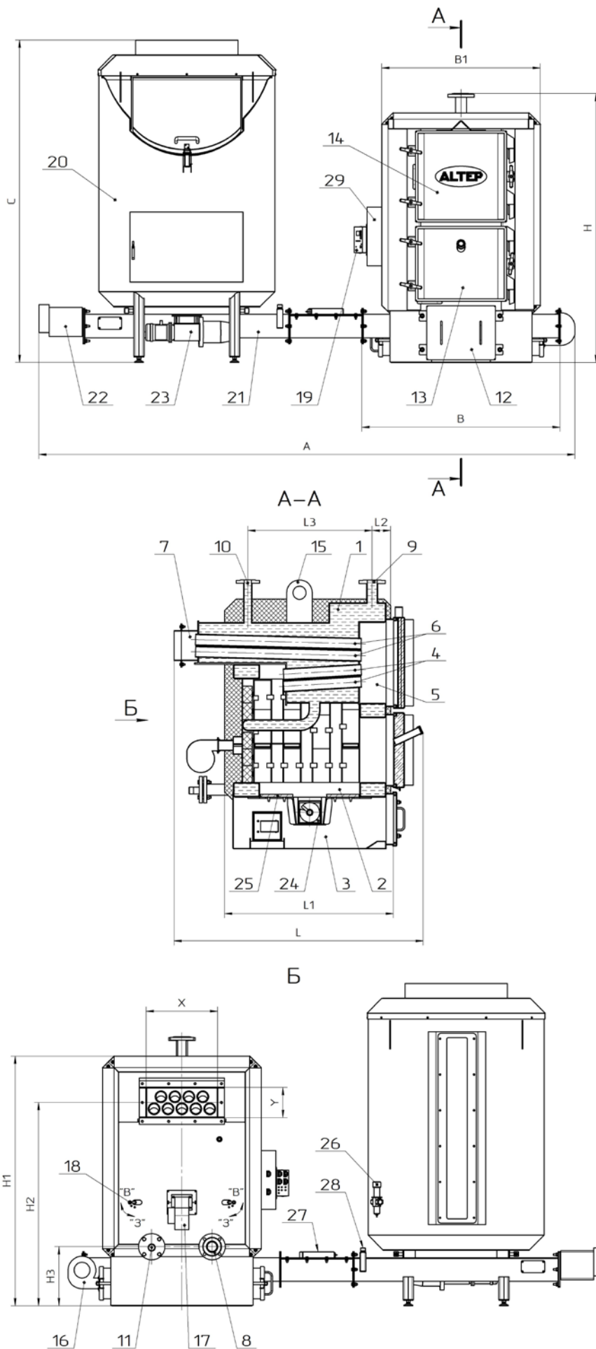
Рисунок 1 – Зовнішній вигляд та основні елементи котла
