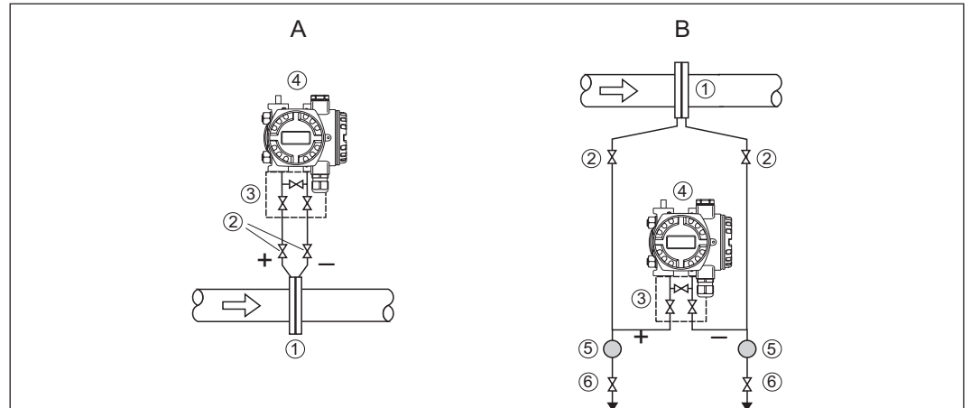
A: предпочтительная конфигурация; B: альтернативная конфигурация (на случай невозможности установки преобразователя над трубой) 1: плоская диафрагма; 2: отсечные клапаны; 3: трехвентильный блок; 4: преобразователь перепада давления Deltabar; 5: сепаратор; 6: спускные вентили
