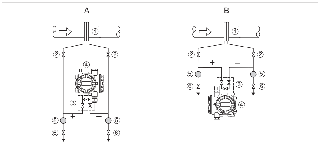
A: предпочтительная конфигурация; B: альтернативная конфигурация (меньшие установочные размеры; только для чистых продуктов) 1: плоская диафрагма; 2: отсечные клапаны; 3: трехвентильный блок; 4: преобразователь перепада давления Deltabar; 5: сепаратор; 6: спускной ventиль
