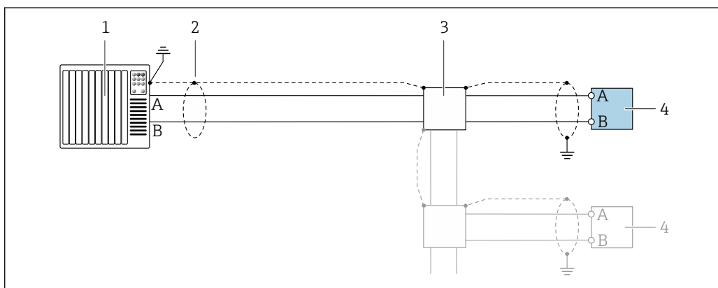
6 Пример подключения для Modbus RS485, безопасная зона и зона 2/разд. 2
