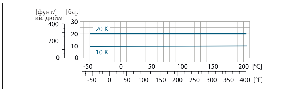
20 С материалом фланца 1.4301 (304); смачиваемые части: цирконий 702, тантал
