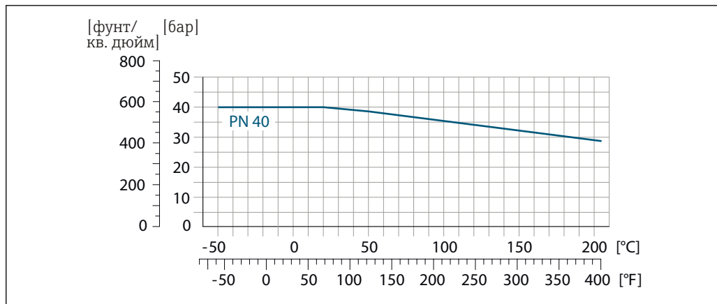
18 С материалом фланца 1.4301 (304); смачиваемые части: цирконий 702, тантал
