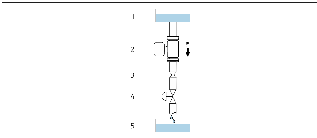
16 Монтаж в трубе с нисходящим потоком (например, для дозирования)
