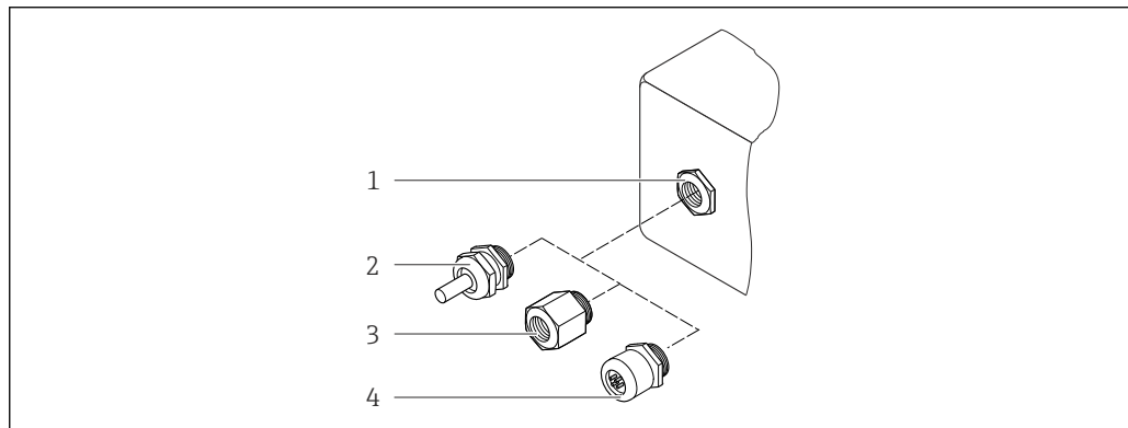
25 Доступные кабельные вводы/кабельные уплотнители
