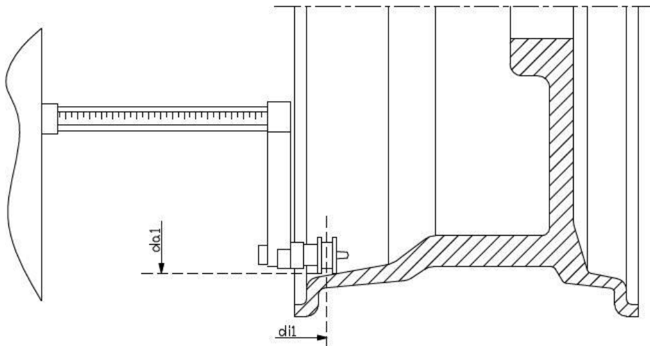
Рисунок 3.8 - Автоматическое получение расстояния к внутренней плоскости в Типе программы als2
