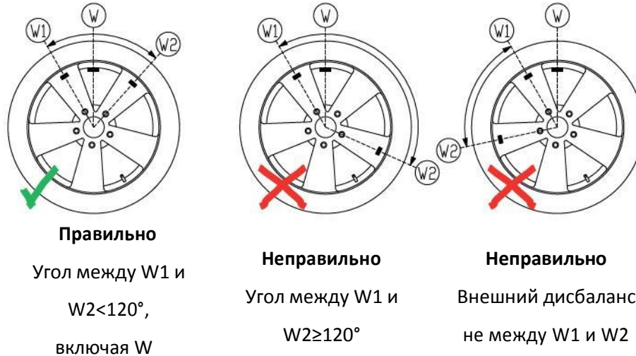
Рис.6.1 – Правильное и неправильное расположение скрытых грузиков
