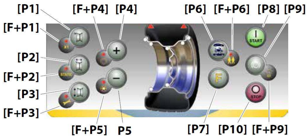
Рисунок 1b – Нумерация вторичных функций кнопок
