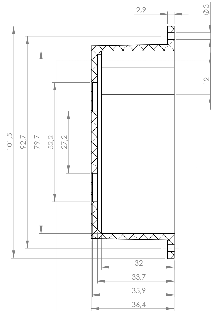
PRZEKRÓJ A-A
