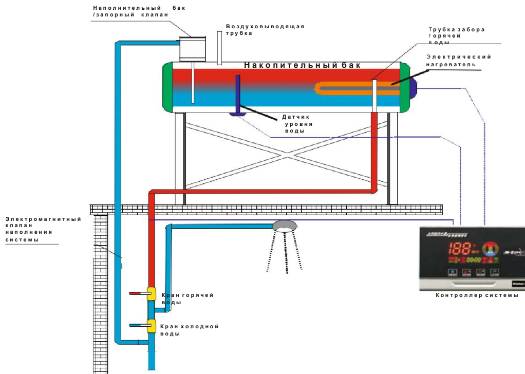
Рис. 2.2 Схема безнапорной системы с механическим наполнением бака
