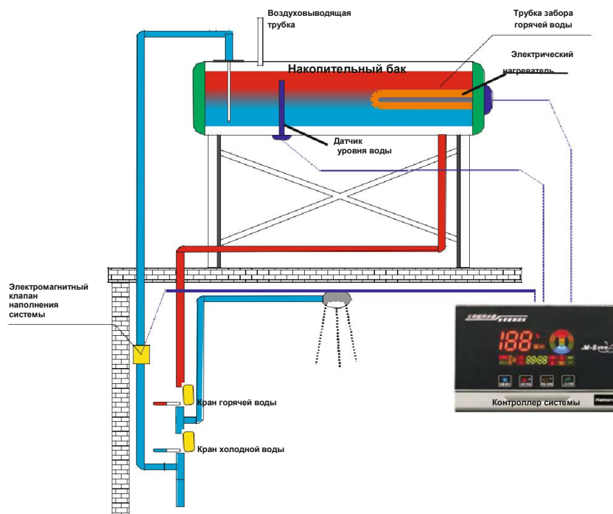
Рис. 2.3 Схема безнапорной системы с электронным наполнением бака
