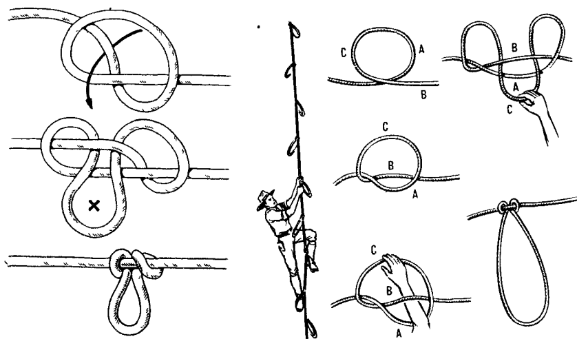
▲ Рис 73 Бурлацкая петля
