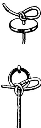
Рис 91 Развязывающийся простой узел
