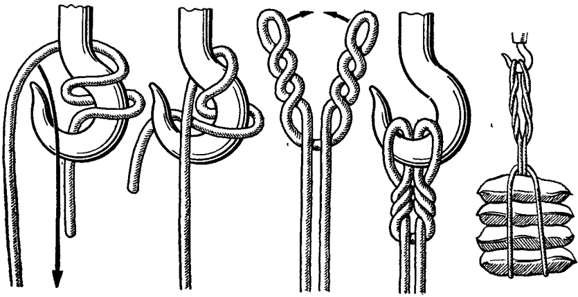
Рис. 106. Гачный узел со шлагом
