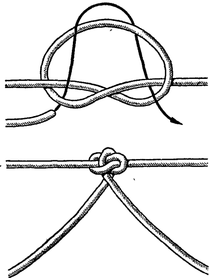
Рис. 130. Поводковый на основе простого узла
