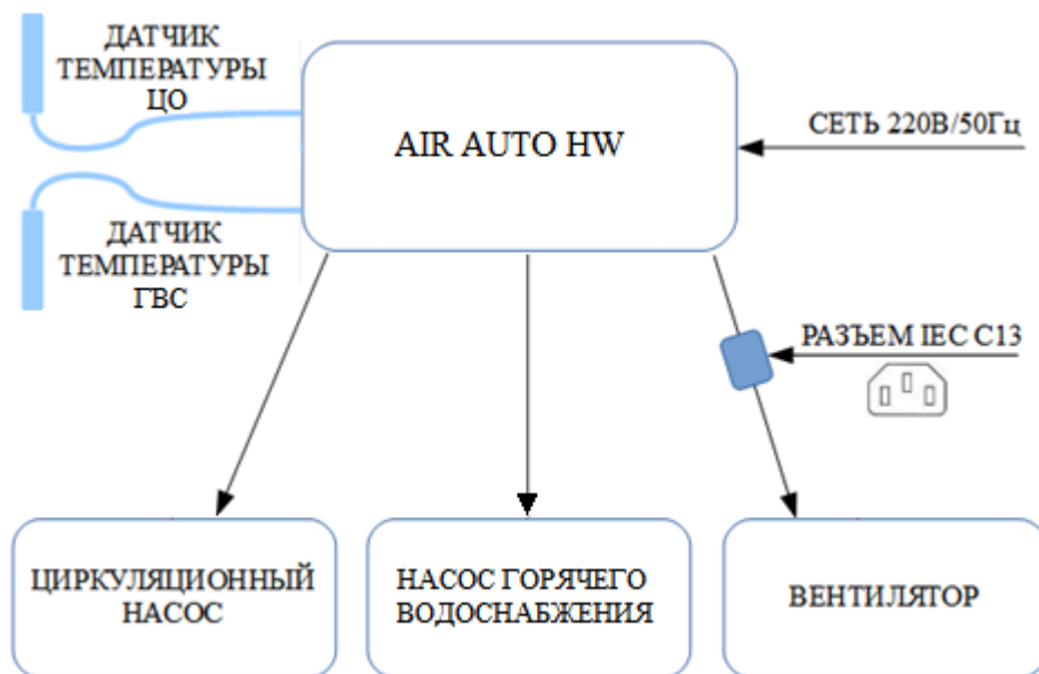
Рисунок 1 – Схема подключений AIR AUTO HW
