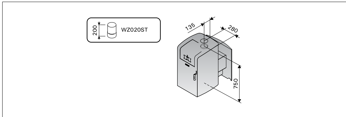
Рисунок 9. Присоединение каменки к каменному дымоходу (все размеры приведены в миллиметрах) Joonis 9. Kerise ühendamise suitsulõõriga (kõik mõõtmised millimeetrites)
