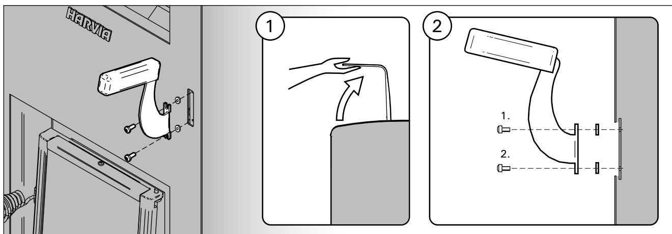
Рисунок 10. Установка рукояток
