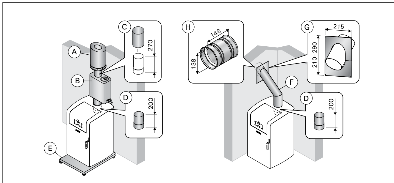
Рисунок 12. Дополнительные принадлежности (все размеры приведены в миллиметрах)
