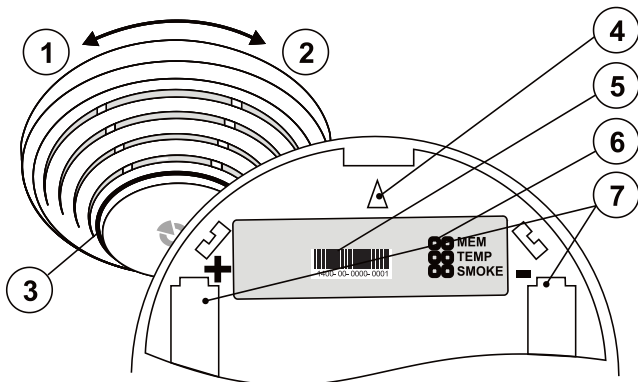
Рис. 6: 1 – открытие крышки детектора; 2 – закрытие крышки детектора; 3 – оптический индикатор состояния; 4 – стрелка, показывающая, куда в нижней части вставлять детектор; 5 – код изделия; 6 – переключки для настройки; 7 – держатели батареек
