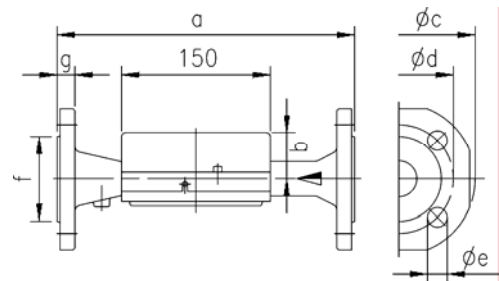
Преобразователи DN25 и DN100 с фланцевым присоединением
