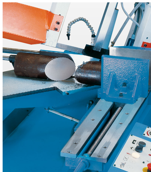
HB 320 BS: автоматический отвод рамы пилы по окончании распила
