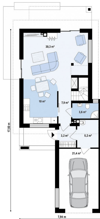
План 1-го этажа
