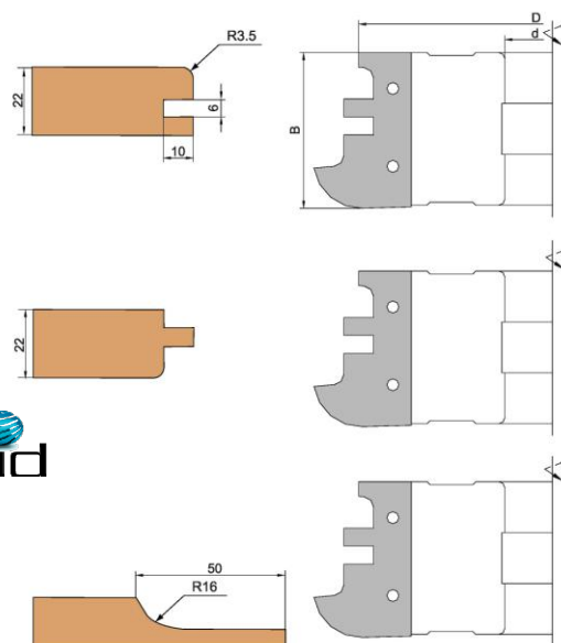
Технические характеристики фрез
