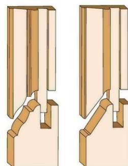
Профиль обработки мебельной обвязки под стекло
