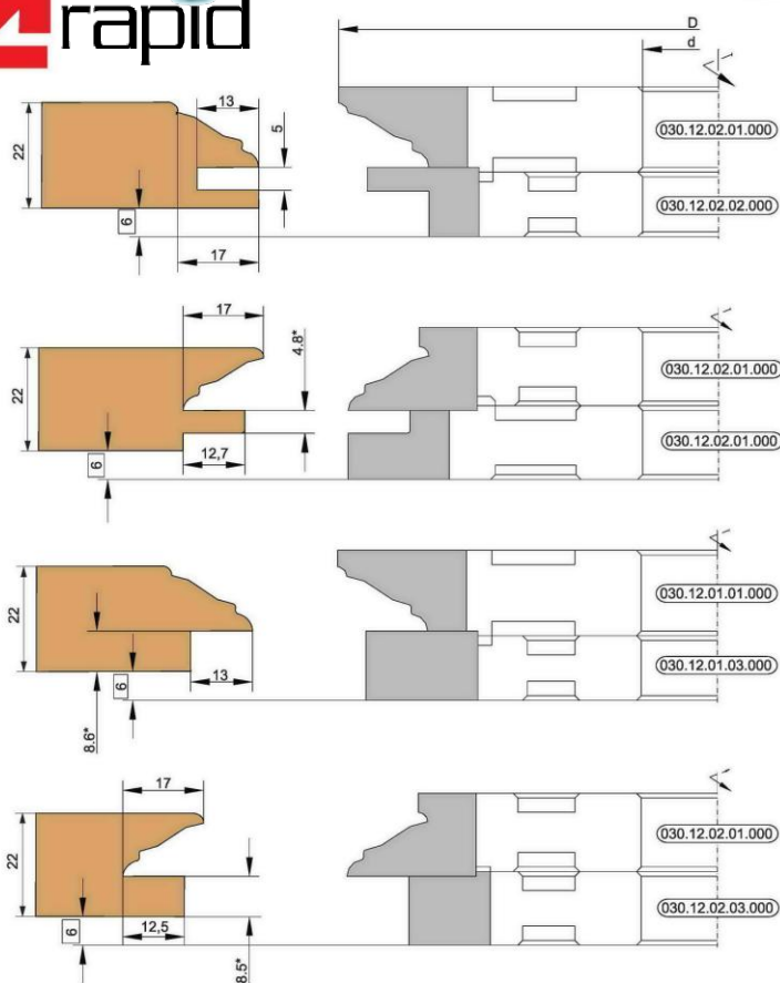
Технические характеристики фрез
