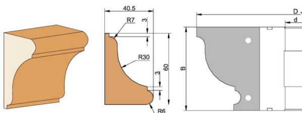
Технические характеристики фрез
