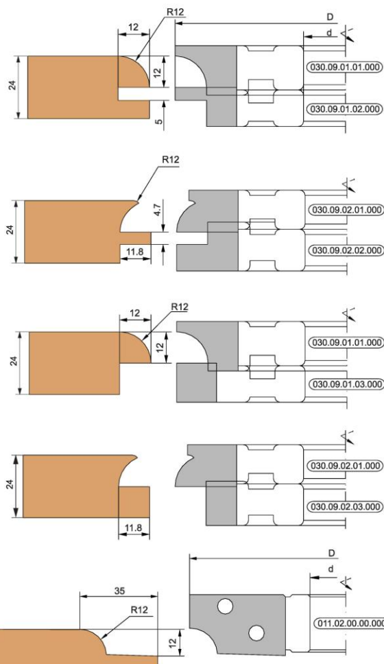
Технические характеристики фрез
