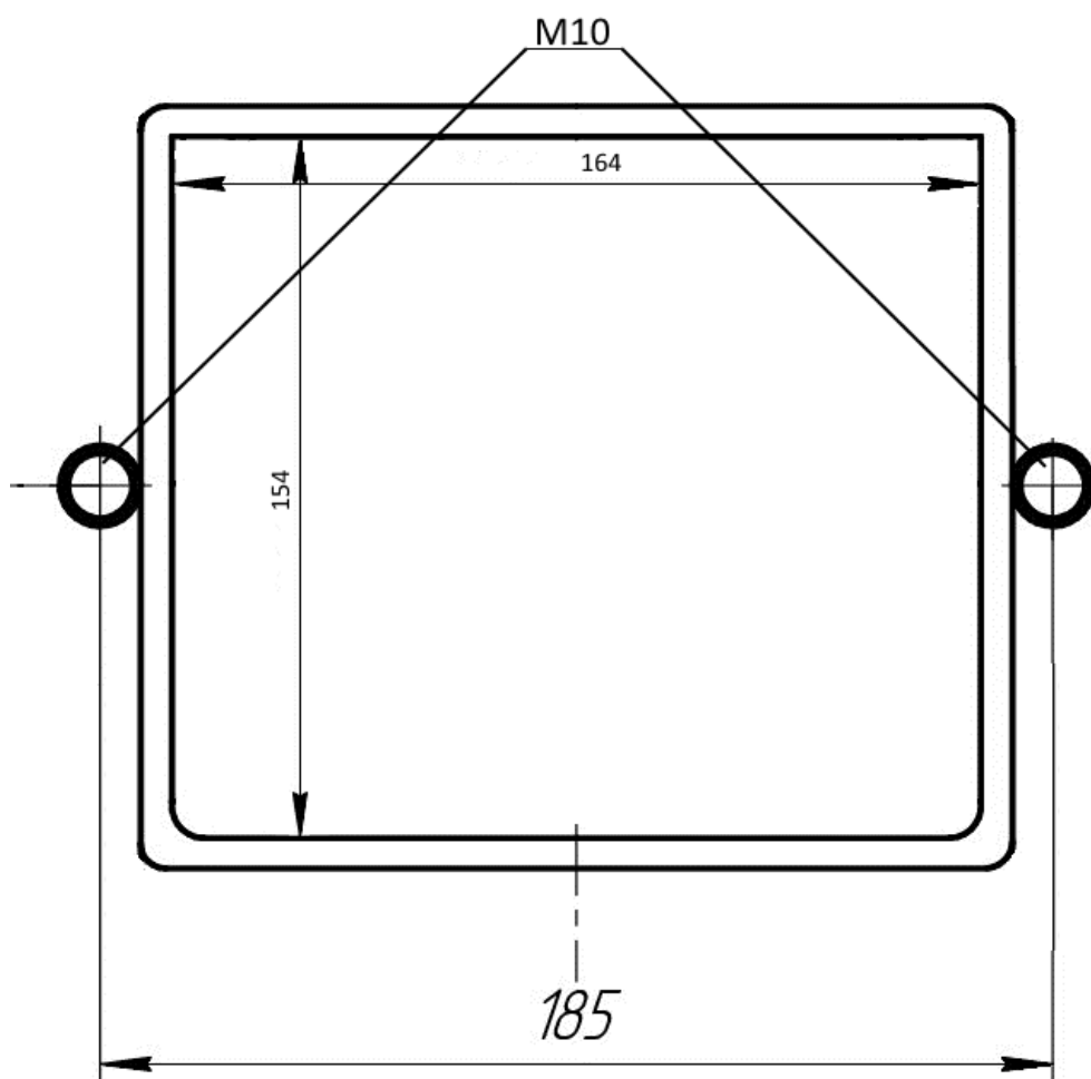
Рис. 4 – Чертеж монтажных отверстий горелки
