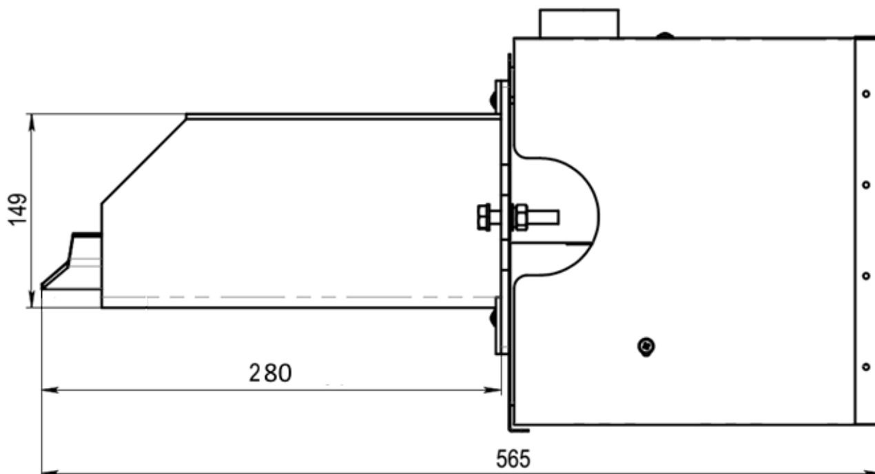
Рис. 3 – Габаритные размеры горелки
