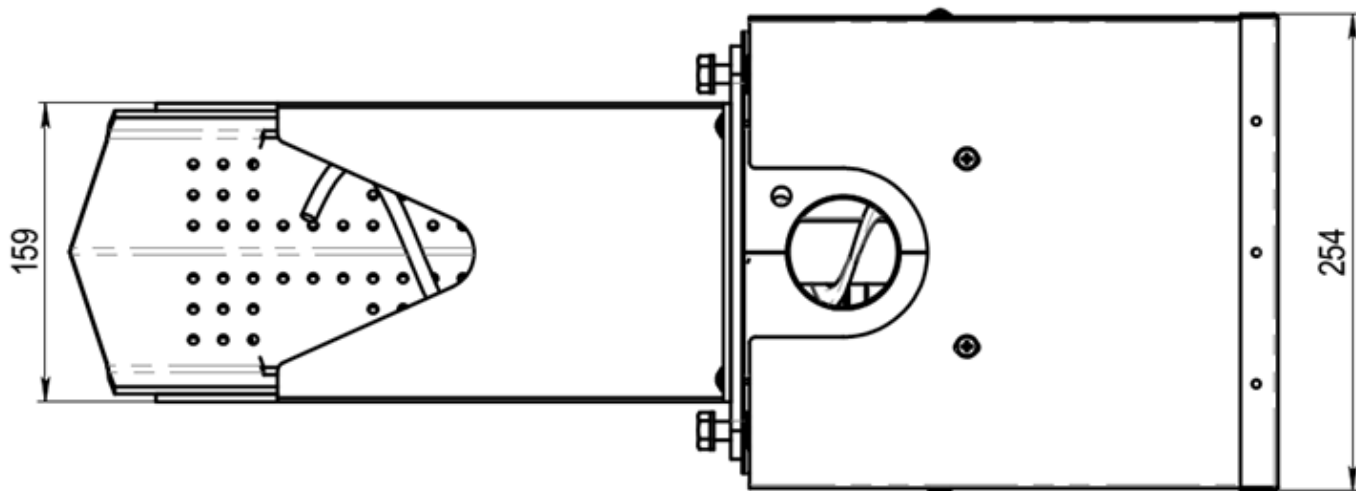
Рис. 3.1– Габаритные размеры горелки
