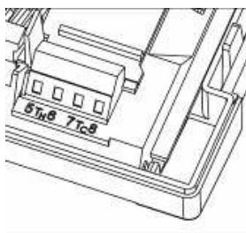
Рис.В Подсоединение датчиков температуры
