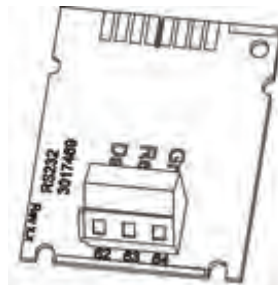
Рисунок J-2 - Модуль RS-232
