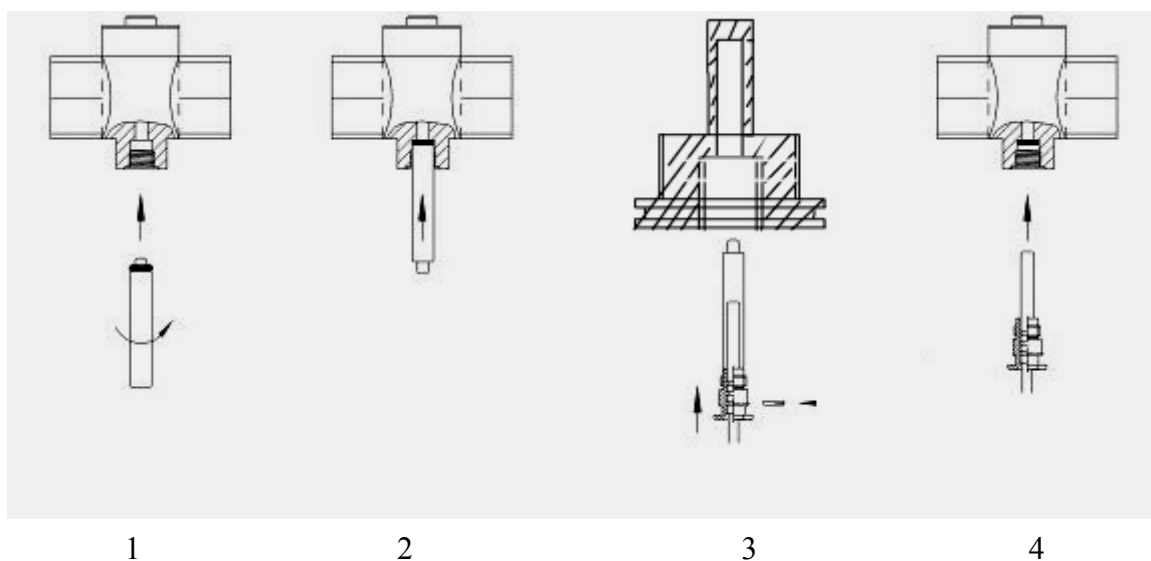
Рисунок М - Монтаж термopеобразователей сопротивления
