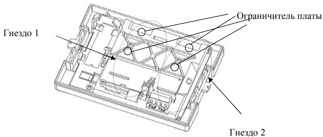
Рисунок H - Монтаж дополнительных модулей в теплосчетчике
