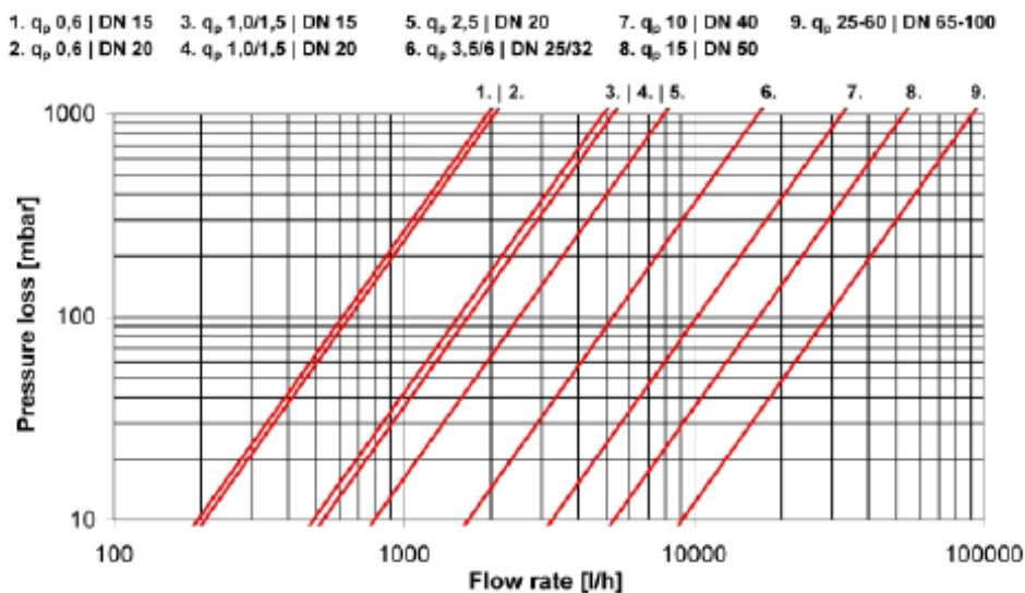
Рисунок 1 - Диаграмма потери давления теплосчетчика SHARKY
