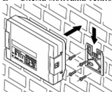
Рисунок F - Схема настенного монтажа вычислителя
