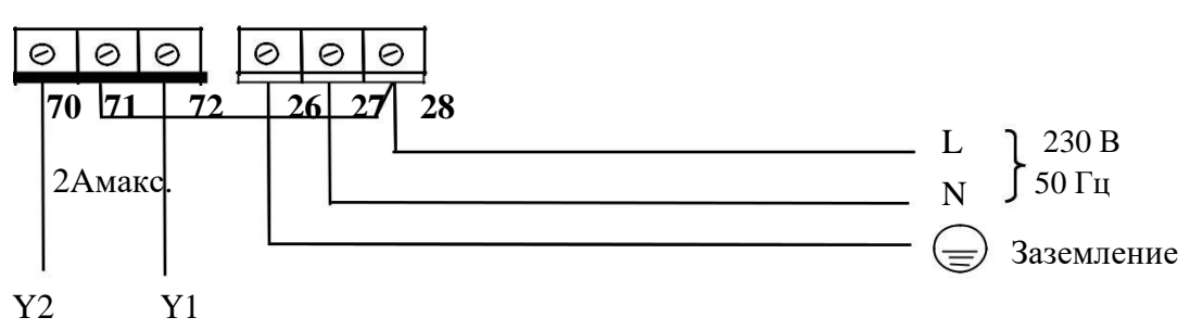
Рис.А4. Схема подключения вычислителя к сети питания переменного тока напряжением 230 В и схема подключения сервопривода к вычислителю (для выполнения функции регулирования) Питание сервопривода и вычислителя от сети переменного тока напряжением 230 В
