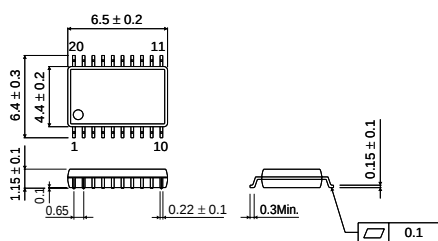
SSOP-B20
