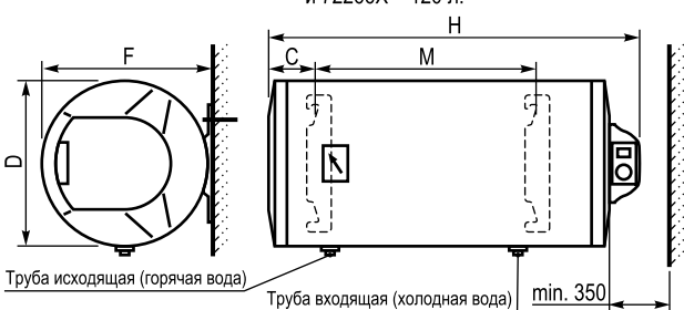
Фиг. 4 Водонагреватели 72265X – 80 л., 72270X – 100 л. и 72266X – 120 л.
