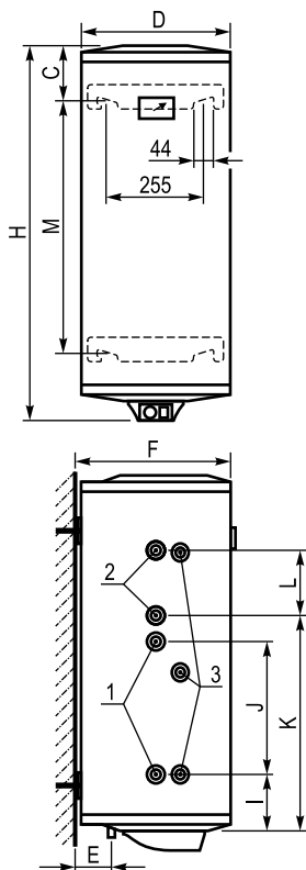
Фиг. 1 Водонагреватели вертикальные, без теплообменника и с теплообменником
