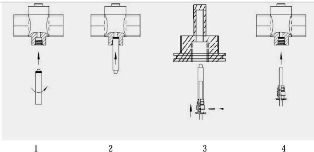
Рисунок М - Монтаж термопреобразователей сопротивления
