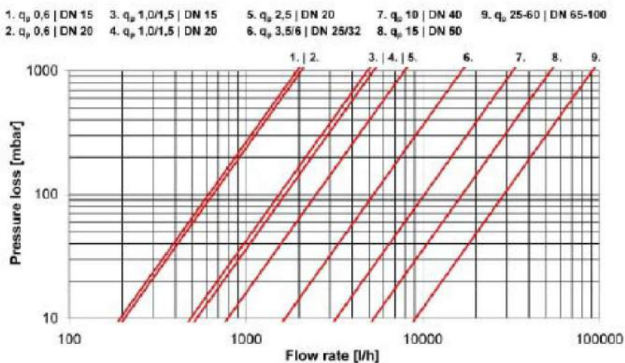
Рисунок 1 - Диаграмма потери давления теплосчетчика SHARKY
