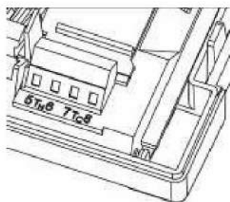
Рис.В Подсоединение датчиков температуры
