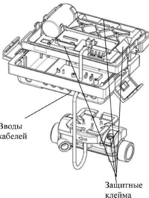
Рисунок С - Схема монтажа термопреобразователей сопротивления
