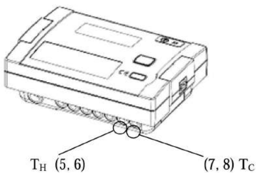
Рисунок D - Схема монтажа термопреобразователей сопротивления
