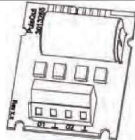
Рисунок К-2 - Модуль импульсных выходов
