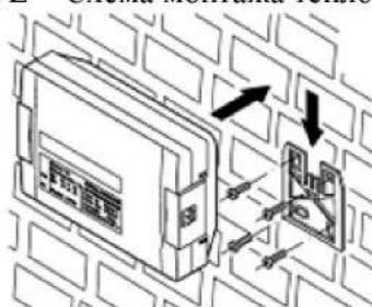
Рисунок Е - Схема монтажа теплосчетчика
