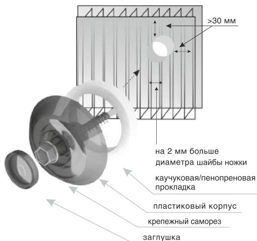
Рисунок 17. Крепление панелей с помощью термошайб.
