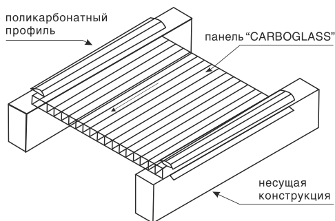
Рисунок 3. Двустороннее крепление.
