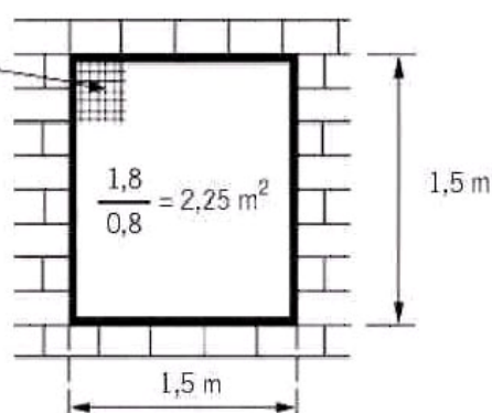
Пример вентиляционного окна с решеткой
