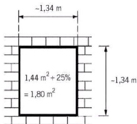
Вентиляционное отверстие в стене
