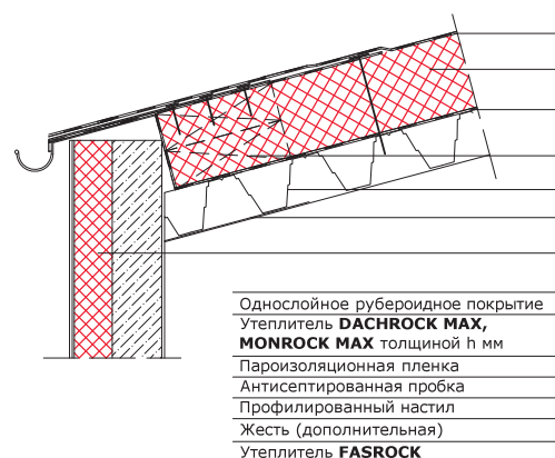
5. Карниз
