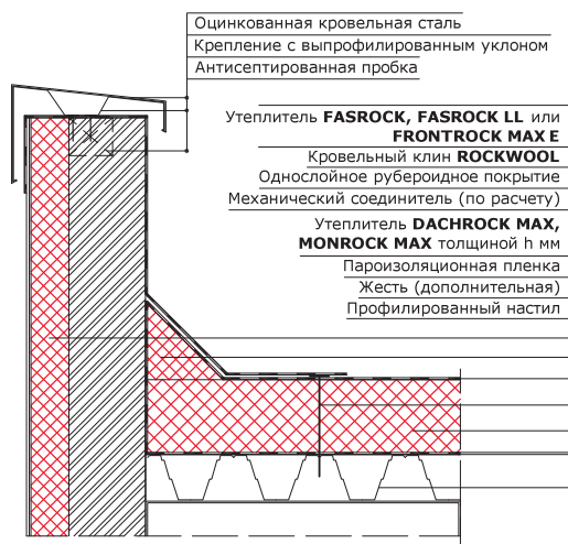
1. Парапетная неветилируемая стена
