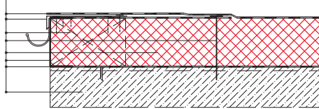
6. Карниз
