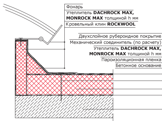
4. Основание фонаря
