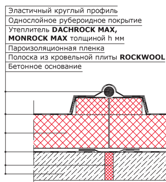
5. Деформационный шов
