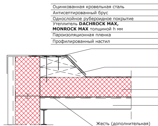
6. Низкий парапет
