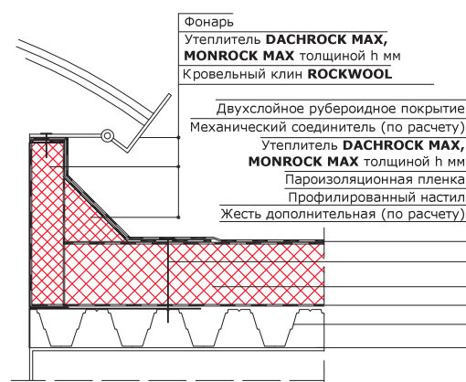
4. Основание фонаря
