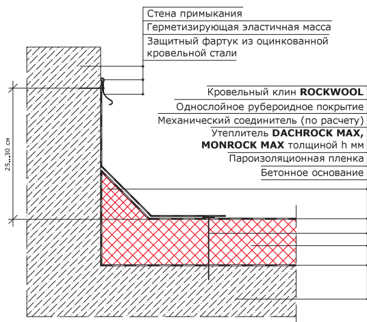
2. Примыкание к стене
