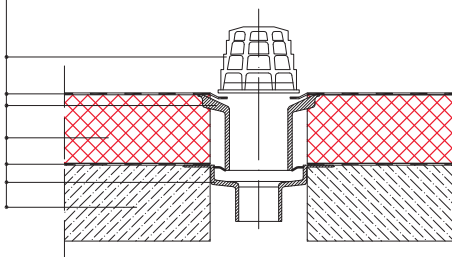
3. Кровельная водоприемная воронка
