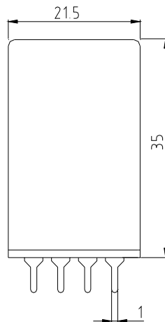
PCB Terminal 印刷线路板式
