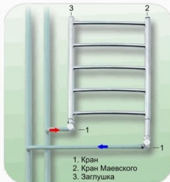
2. Нижнее подключение
