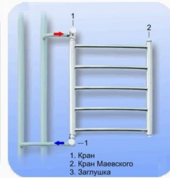
3. Прямое подключение
