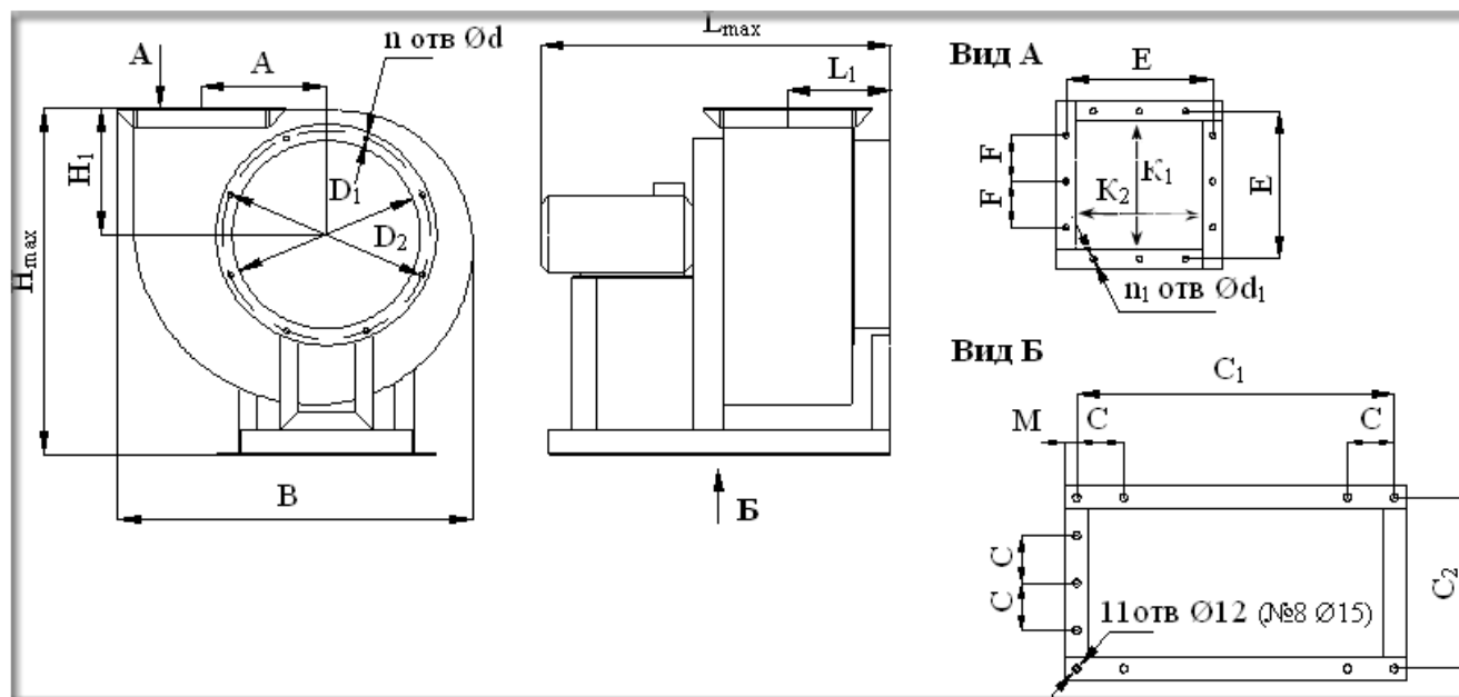
Габаритные размеры
