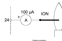
С электродом ионизации
