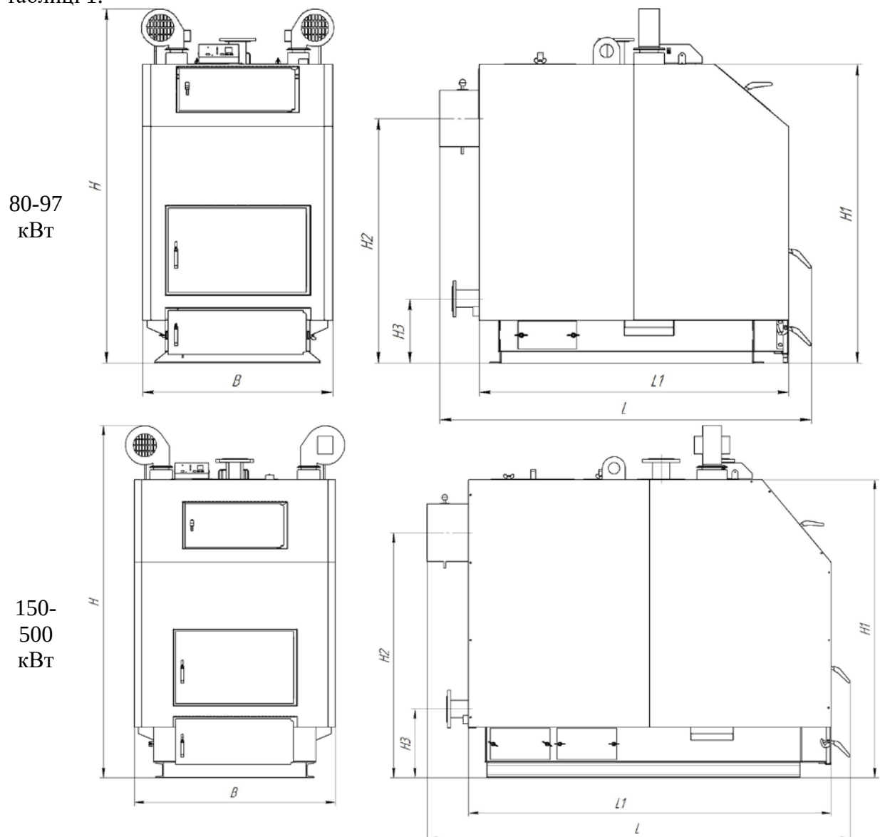
Рисунок 1 – Габаритне креслення котла типу КТ-3-Н
