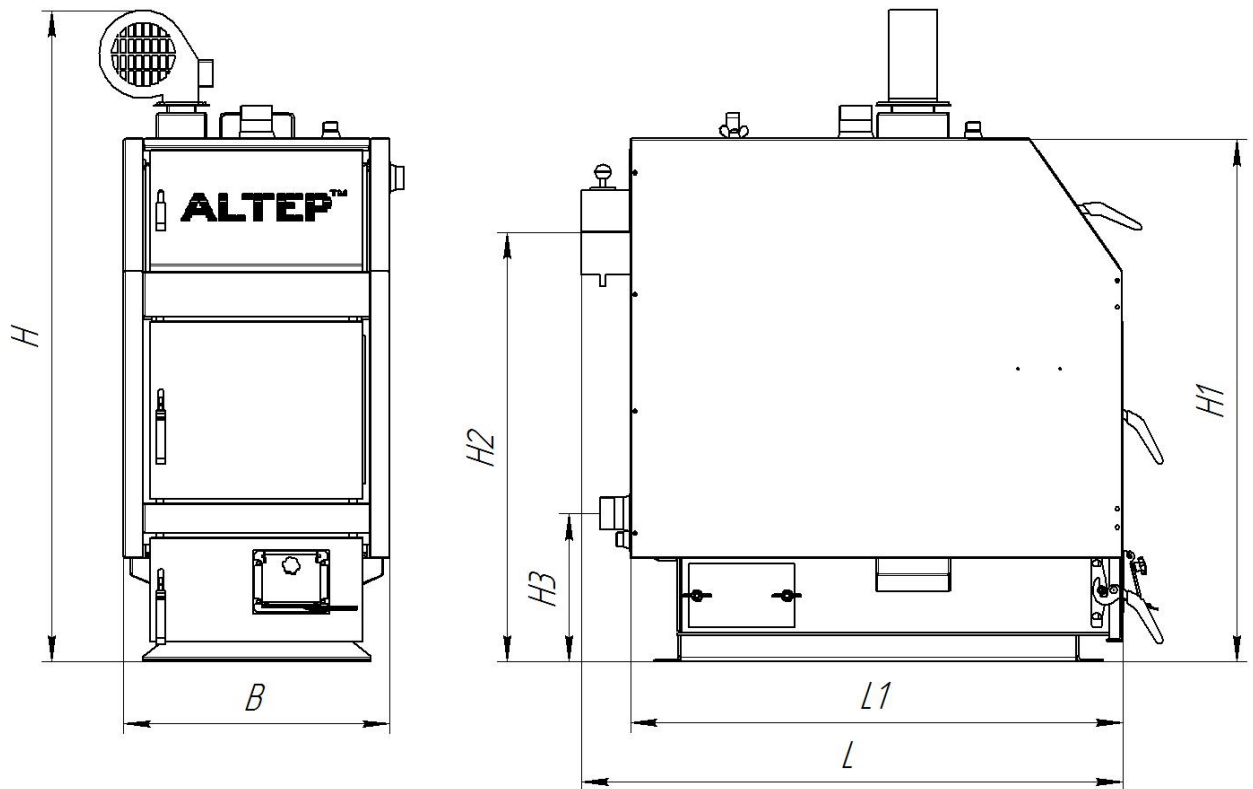
Рисунок 1 – Габаритне креслення котла типу КТ-3-Н
