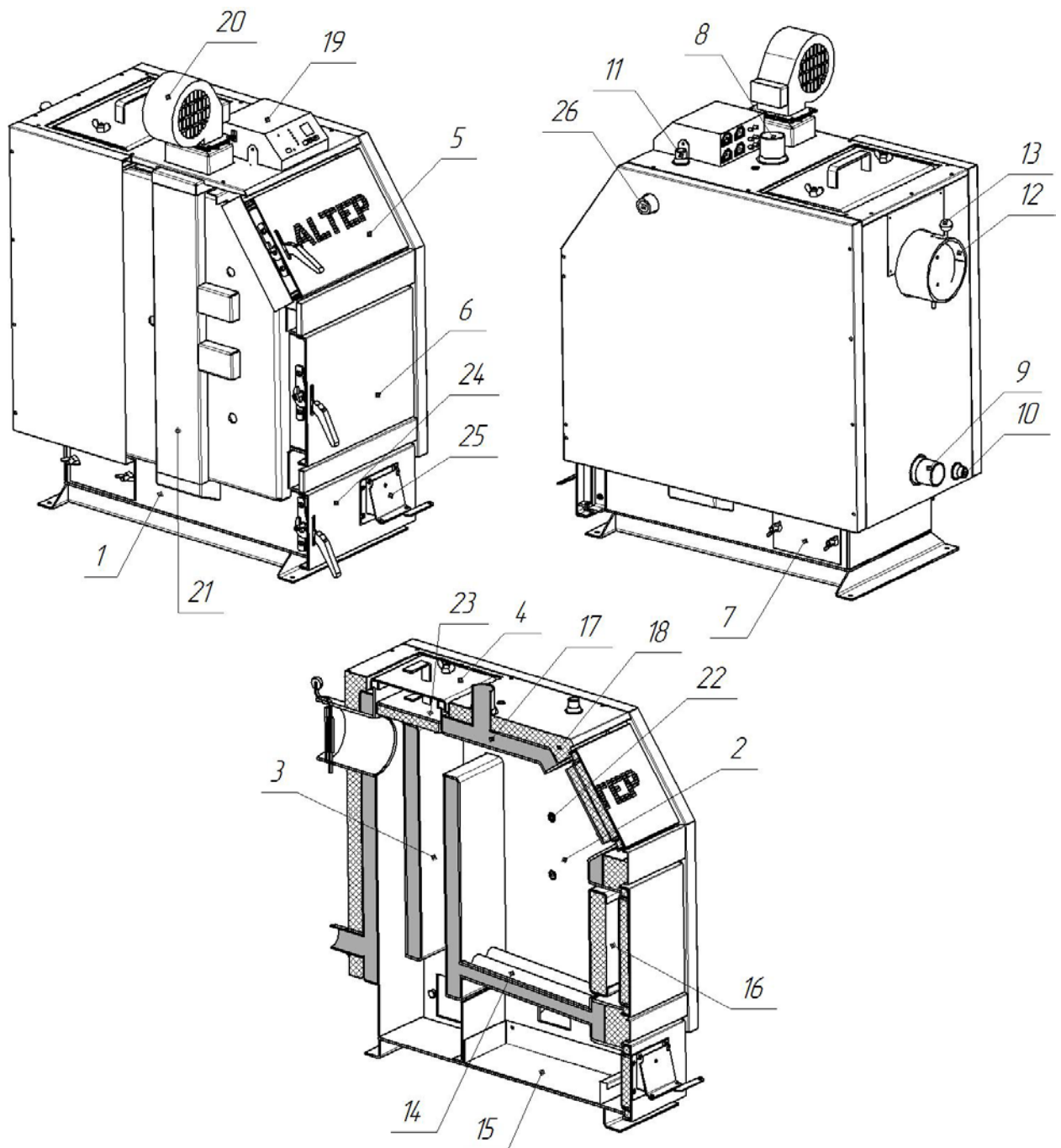
Рисунок 2 – Зовнішній вигляд та основні елементи котла
