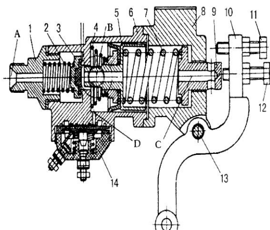
Рис. 5-25 Тормозной клапан
