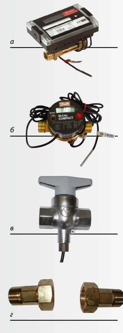
Рис. 11. Теплосчетчики: а — SONOMETR 1000; б — M-Cal Compact 440; в — кран для термопреобразователя; з — соединительные штуцеры.
