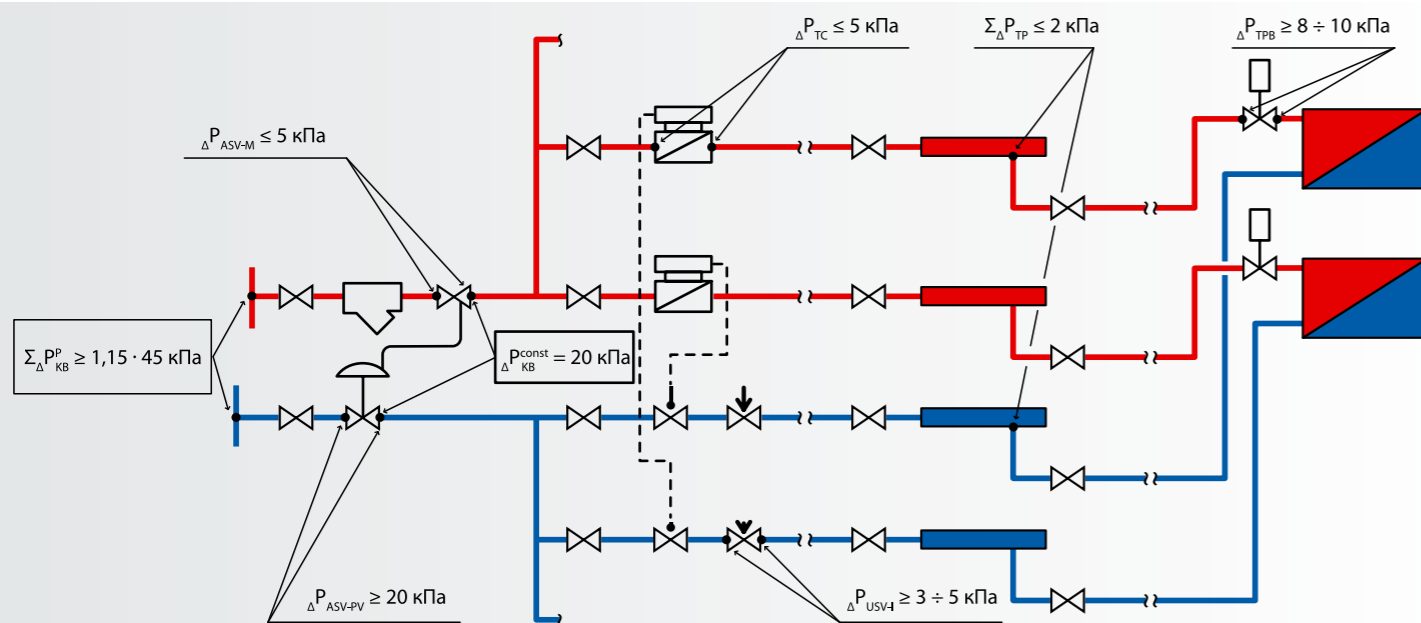
Рис. 21. Пример распределения перепадов давлений в квартирной системе отопления при групповом узле ввода.
