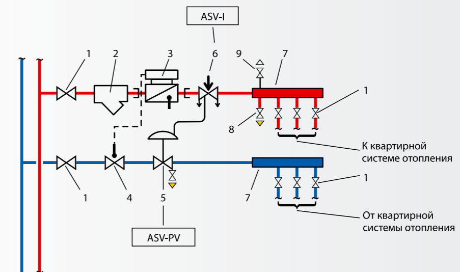
Рис. 8. Принципиальная схема индивидуального квартирного узла ввода.
