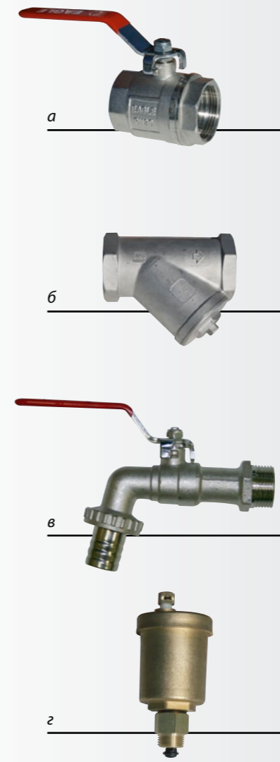
Рис. 10. Трубопроводная арматура: а — шаровый кран; б — сетчатый фильтр; в — спускной кран; з — автоматический воздухоотводчик.
