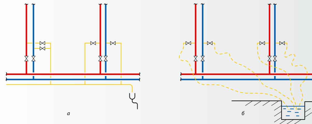
Рис. 5. Устройство дренажа стояков:
