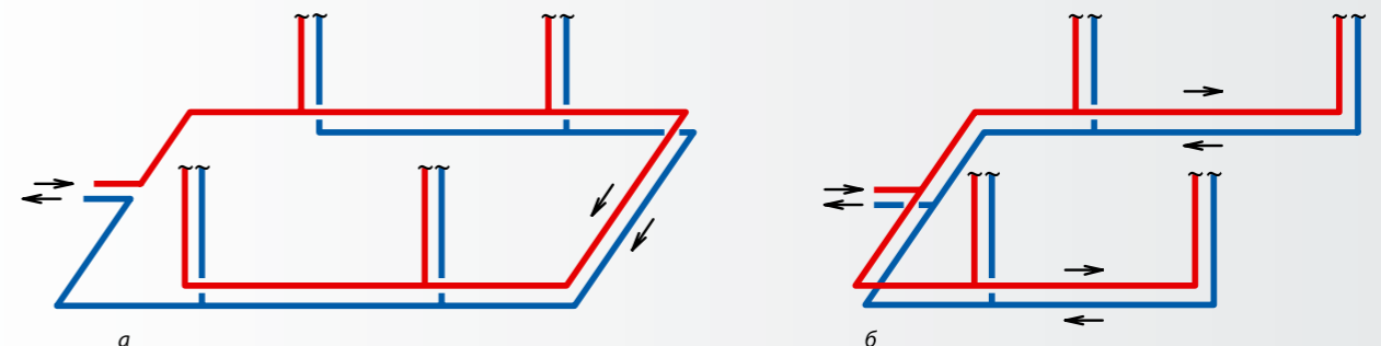
Рис. 3. Направление движения теплоносителя по магистральным трубопроводам: а — однонаправленное (попутное); б — противоточное (тупиковое).
