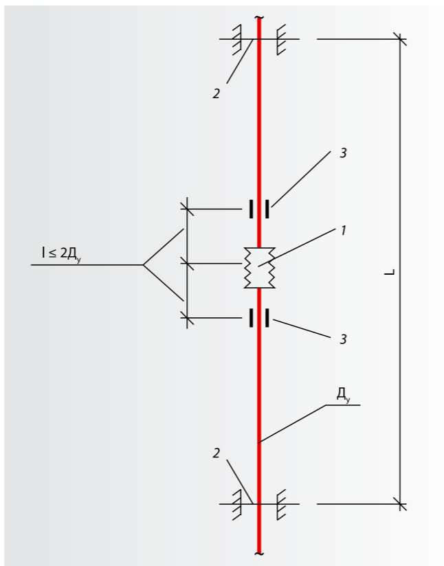
Рис. 6. Установка сильфонных компенсаторов торговой марки HYDRA: 1 — сильфонный компенсатор; 2 — неподвижная опора; 3 — направляющая опора.
