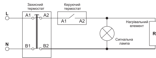
Рис. 10. Схема електрична для моделей Steatite (S3C), (S3S), D400-2-BC, EXPERT, TURBO.
