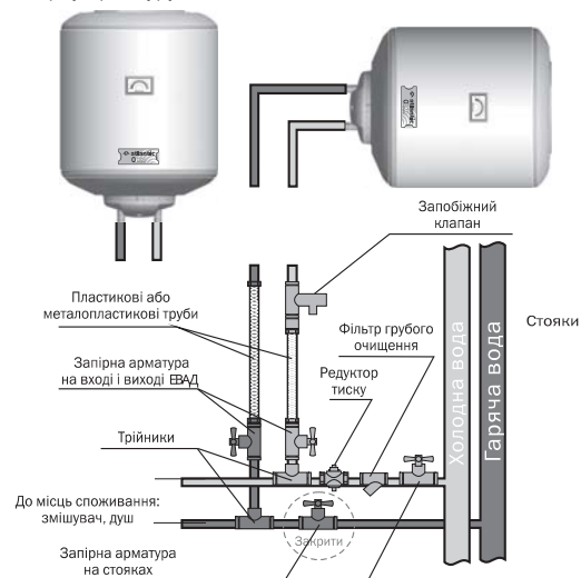
Рис. 5. Підключення ЕВАД у вертикальному / горизонтальному положенні
