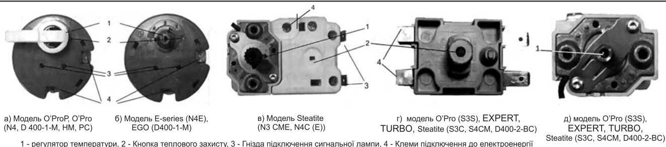
Рис. 3. Зовнішній вигляд терморегулятора
