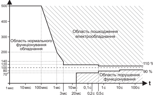
Рис. 1. Крива роботи електрообладнання ITIC (СВEMA), ( http://www.home.agilent.com/upload/cmc_upload/All/1.pdf?&cc=UA&lc=eng ).
