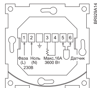
Подключение
