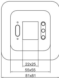
Размеры (мм)
