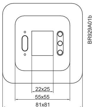
Размеры (мм)
