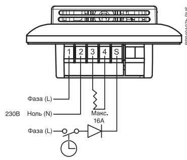
Подключение OTN2-1991
