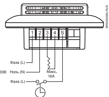
Подключение OTD2-1999 (режим защиты от замерзания)
