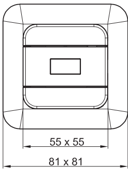
Размеры
