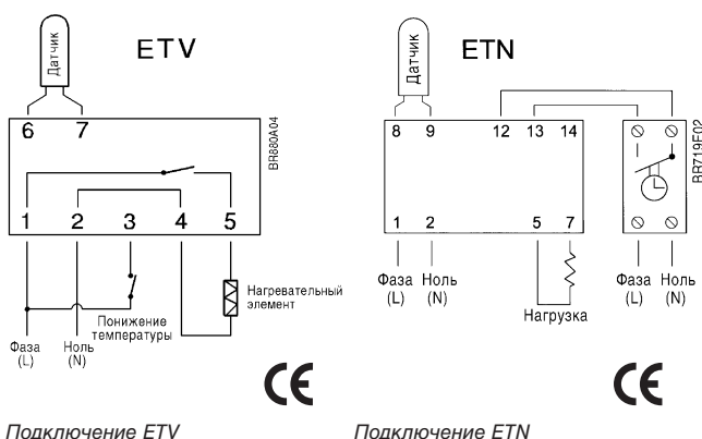
Подключение ETV
