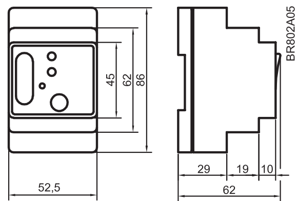
Размеры ETN (мм)
