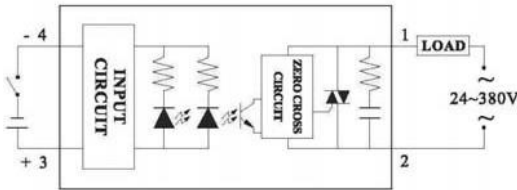
DC-AC тип
