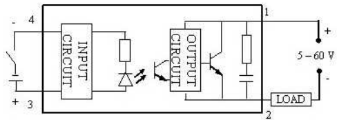
DC-DC тип
