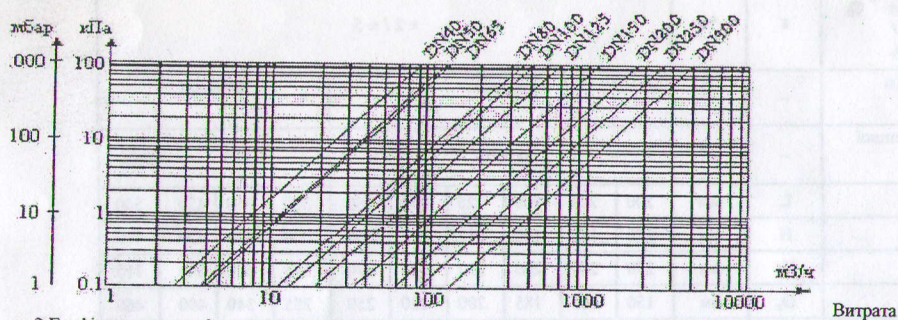
Рис. 2 Графіки залежності втрати тиску від витрати води
