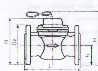
Рис. 1 Лічильник води MWN
