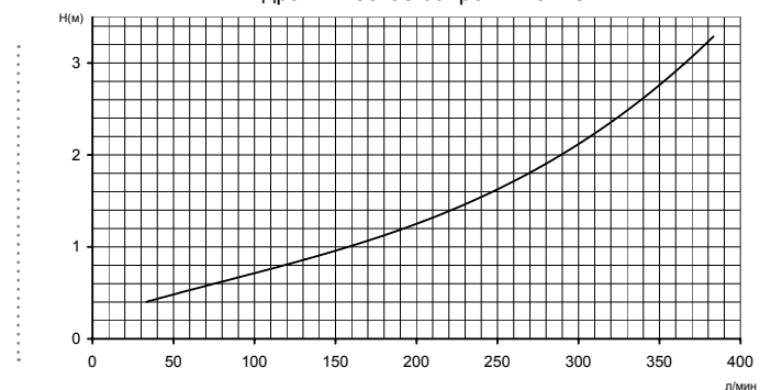
Гидравлическое сопротивление
