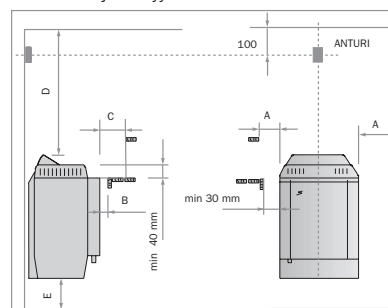
Kiukaan suojaetäisyydet
