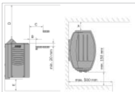
Kiukaan suojaetäisyydet
