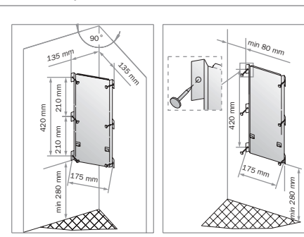
Asennuslevy
