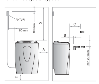
Kiukaan suojaetäisyydet
