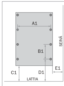
Asennuslevy
