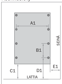
Asennuslevy
