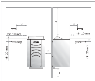
Vega Compact -kiukaan suojaetäisyydet
