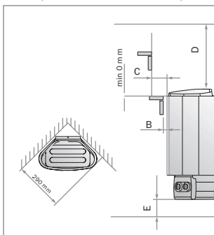
Delta- ja Delta EE -kiukaan suojaetäisyydet
