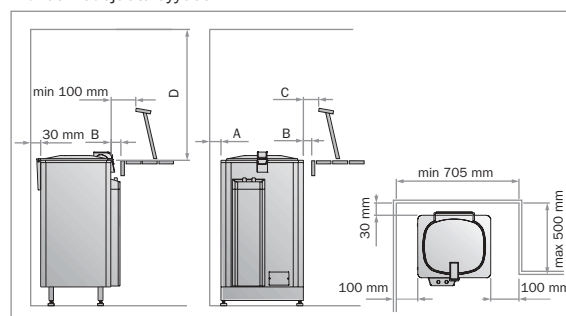
Kiukaan suojaetäisyydet
