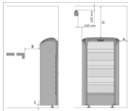
Kiukaan suojaetäisyydet
