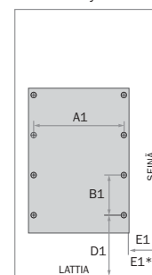
Asennuslevy
