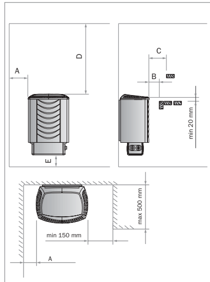
Kiukaan suojaetäisyydet
