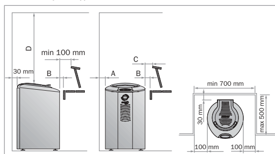
Kiukaan suojaetäisyydet
