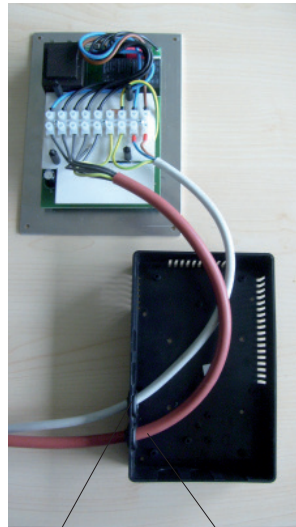
Durchführung für Netzleitung Durchführung für Lampenleitung
