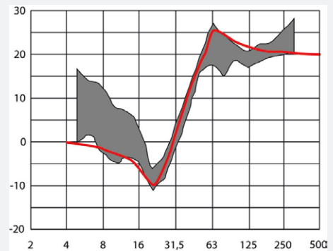
Снижение вибрации при установке здания на упругие опоры из материала Sylomer®
