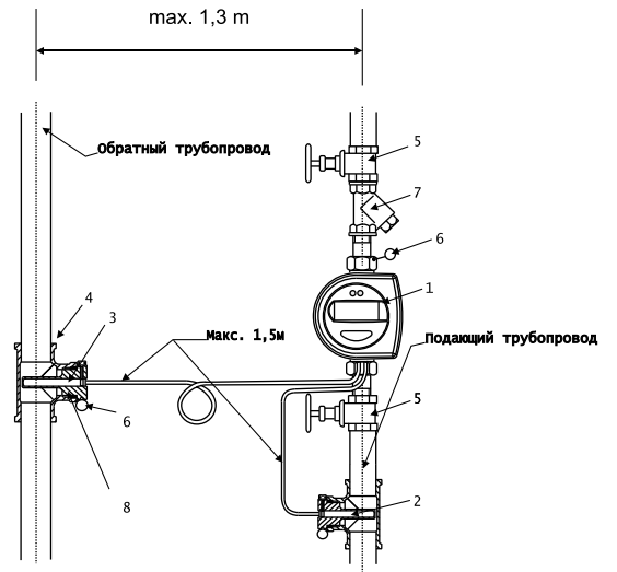
Рис. 3 Монтаж счетчика тепла в вертикальном трубопроводе.
