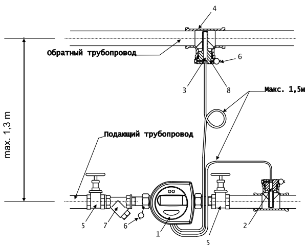
Рис. 4 Монтаж счетчика тепла в горизонтальный трубопровод. Счетчик тепла повернут на 90°С
